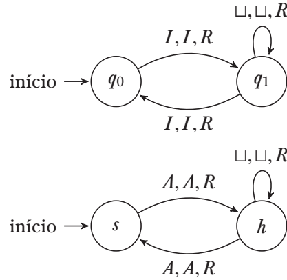
Figura 15.1: Variantes da máquina Par
