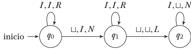
Figura 14.3: Uma máquina que computa f(x, y) = x + y
